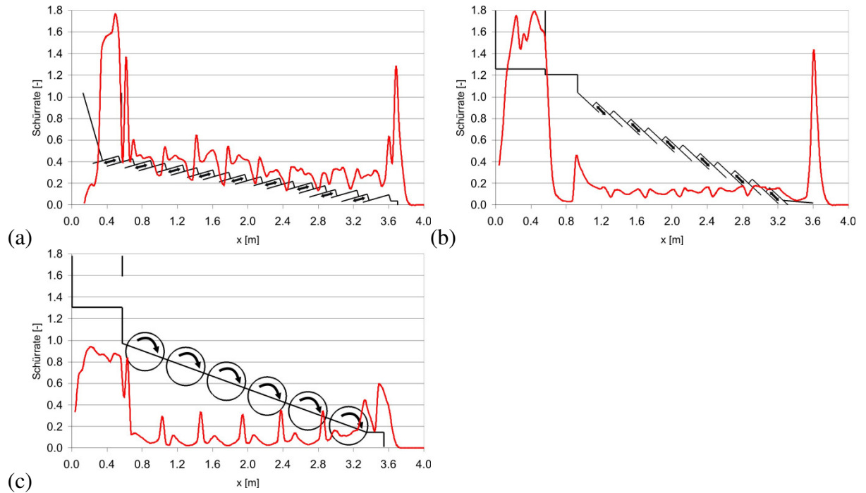
Schürratenverläufe für (a) Vorschub-, (b) Rückschub- und (c) Walzenrost
